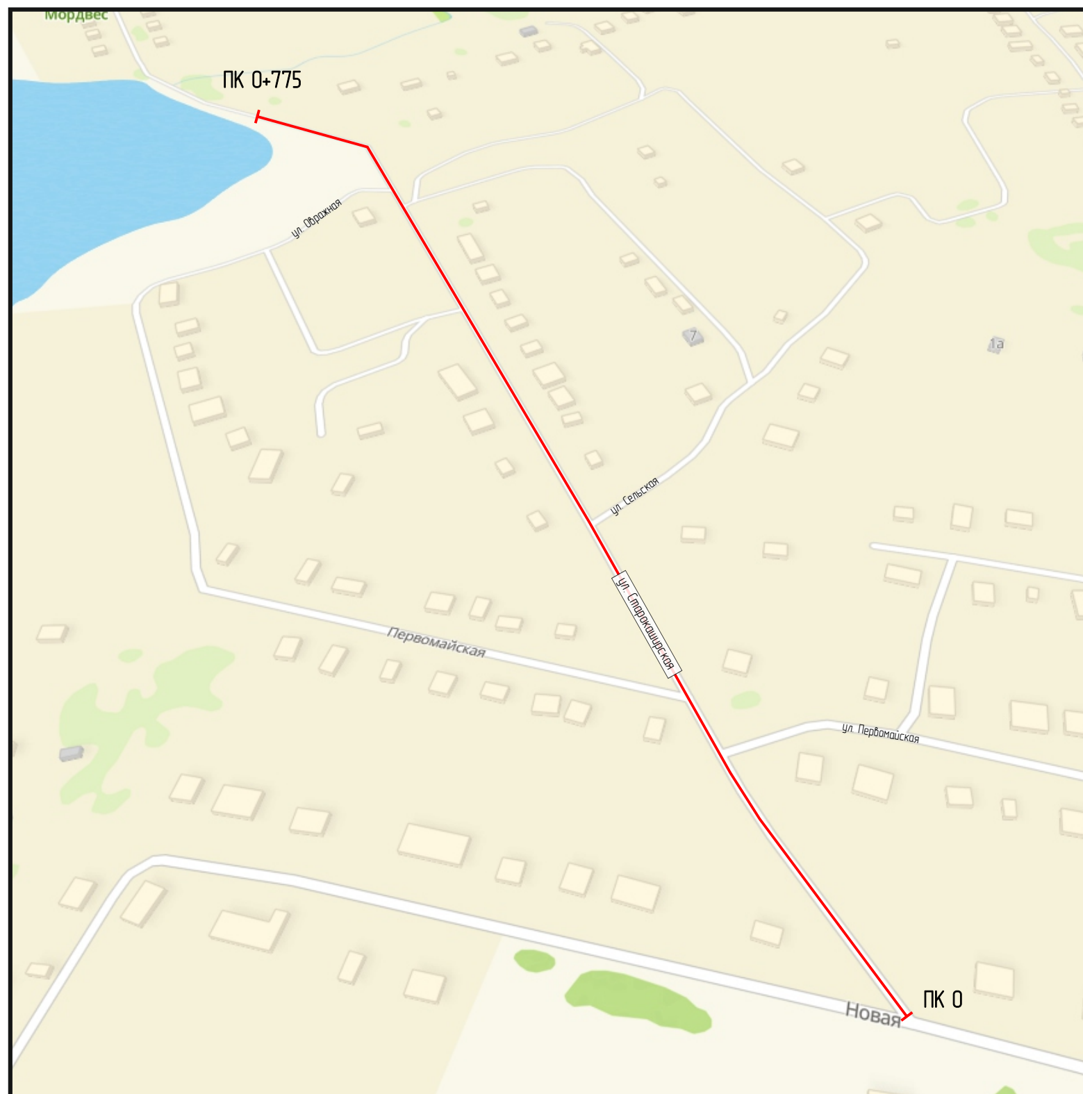
Рис.1 – ситуационный план
